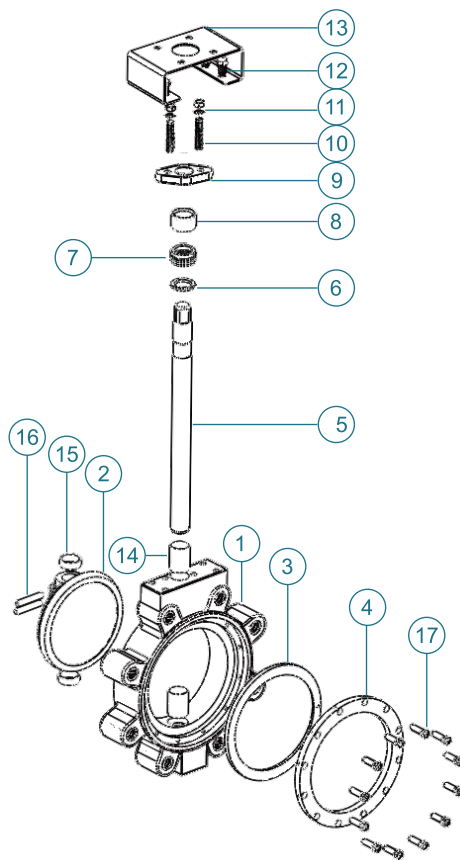
Lug type
